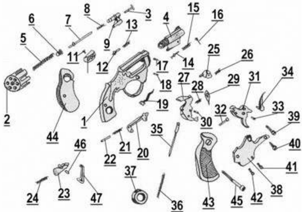
FOTO 50 DETALLE DE LAS PARTES DE UN REVOLVER
