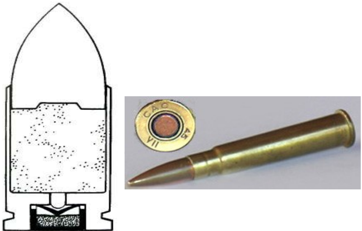
FIGURA 26 ESQUEMA Y CARTUCHO DE FUEGO CENTRAL
