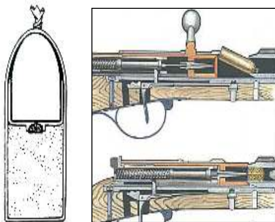
FIGURA 20 CARTUCHO Y FUSIL DE AGUJA DREYSE
