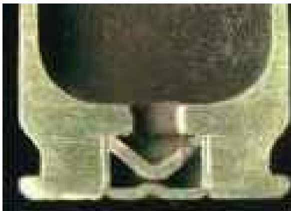
TIPO BOXER YUNQUE INCORPORADO A LA CAPSULA
