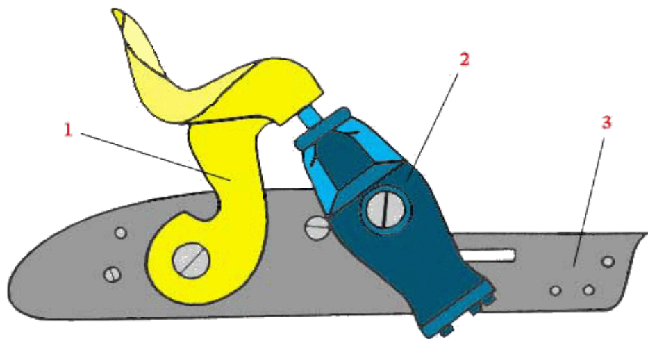
FOTO 19 FRASCO DE PERFUME DE FORSYTH 1- MARTILLO, 2- FRASCO CON INICIADOR, 3- SOPORTE
